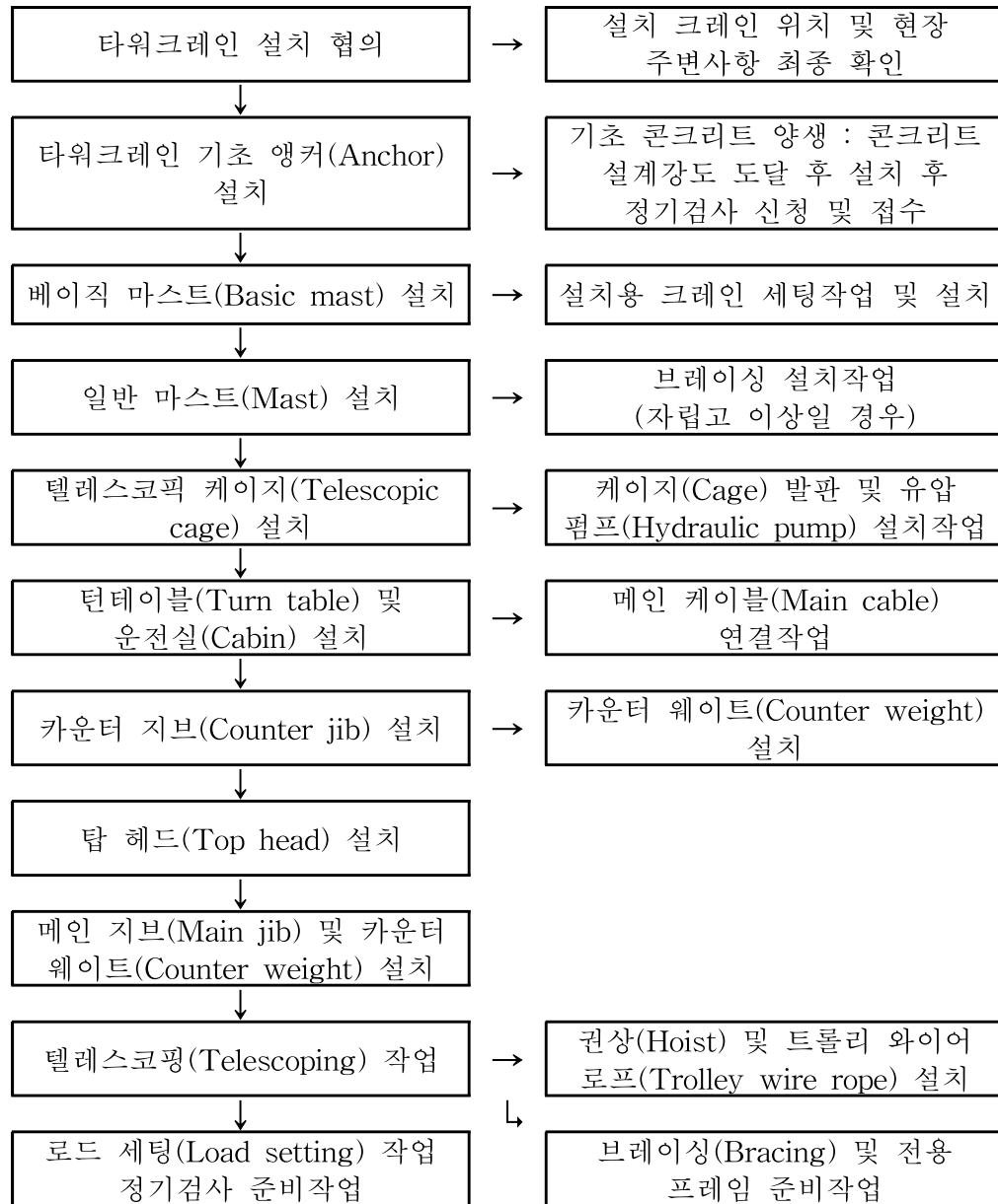
〈그림 6〉 타워크레인 설치·조립작업 흐름도
