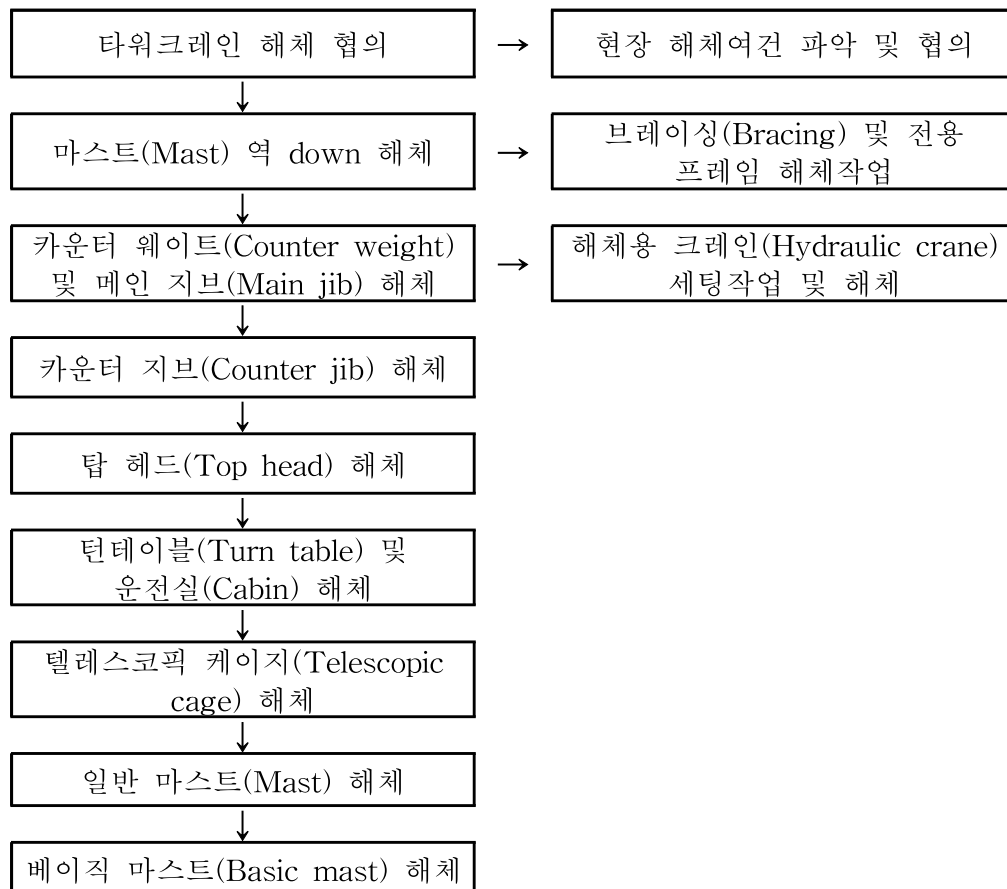
<그림 8> 타워크레인의 해체작업 흐름도
